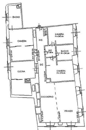
PIANO SECONDO
