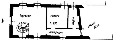
piano primo
