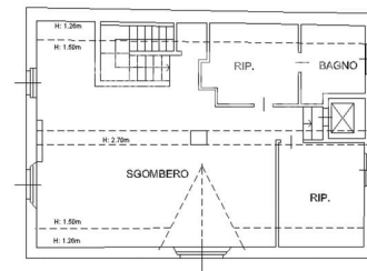
PIANO TERZO (sottotetto)
