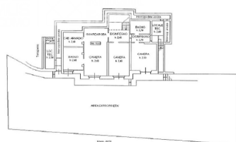
PIANO TERZO SOTTOSTRADA
