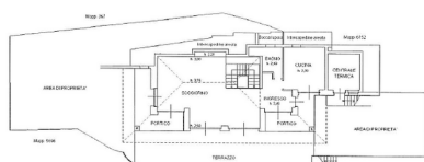
PIANO SECONDO SOTTOSTRADA
