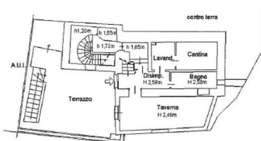
PIANO TERRA h. 2,52m
