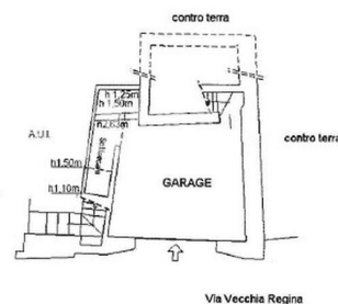
PIANO PRIMO SOTTOSTRADA h. 3,22m
