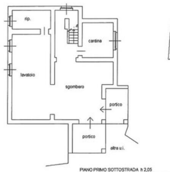
PIANO PRIMO SOTTOSTRADA h 2,05
